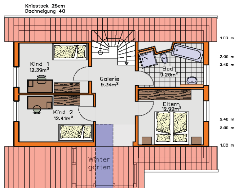
Grundriss DG mit Wintergarten 51 m 2
